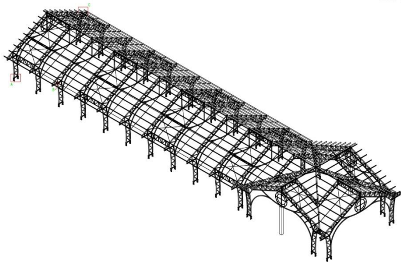
Figura 1.2 – Projeto Isométrico
