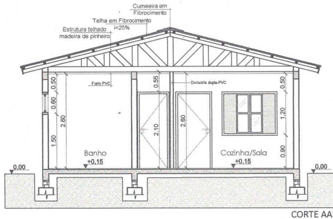
CORTE AA'
