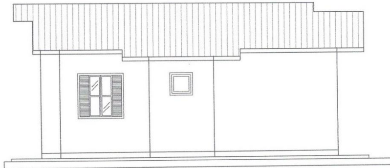
FACHADA LATERAL
