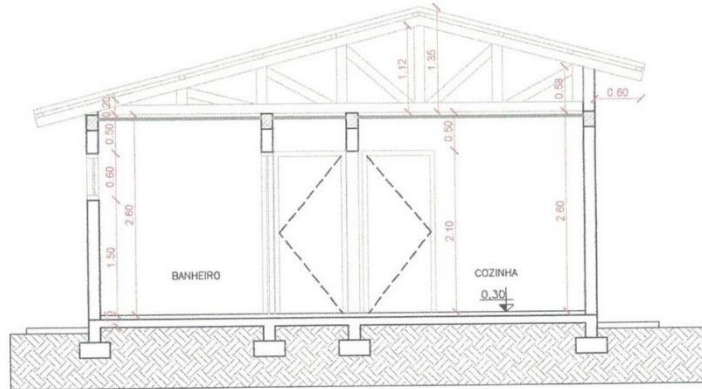
CORTE AA
